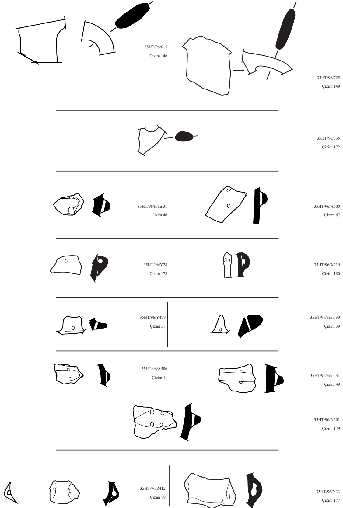
Hüyüktepe - Survey Handle 12, Handle 14, Knob 1, Knob 2, Knob handle 5, Knob handle 6, Bar handle 2, Lug 3A, Lug 3B (M 1:2)
